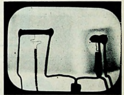
De transistors gezien door dezelfde opneembuis, nu echter bestraald met röntgenstralen, zodat een röntgen-schaduwbeeld is ontstaan.
